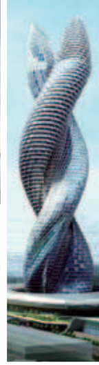
الشكل 01: تطور فكر الحركة بالنسبة لمفهوم الزمن، من حركة ستاتيكية معدل التغير فيها صفر وصولاً إلى حركة ديناميكية عالية
