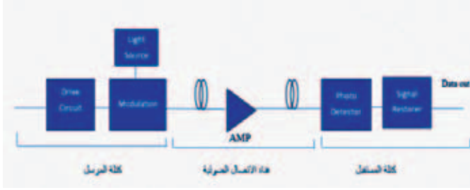
الشكل (3): مخطط صندوق لمكونات نظام الاتصالات البصري
